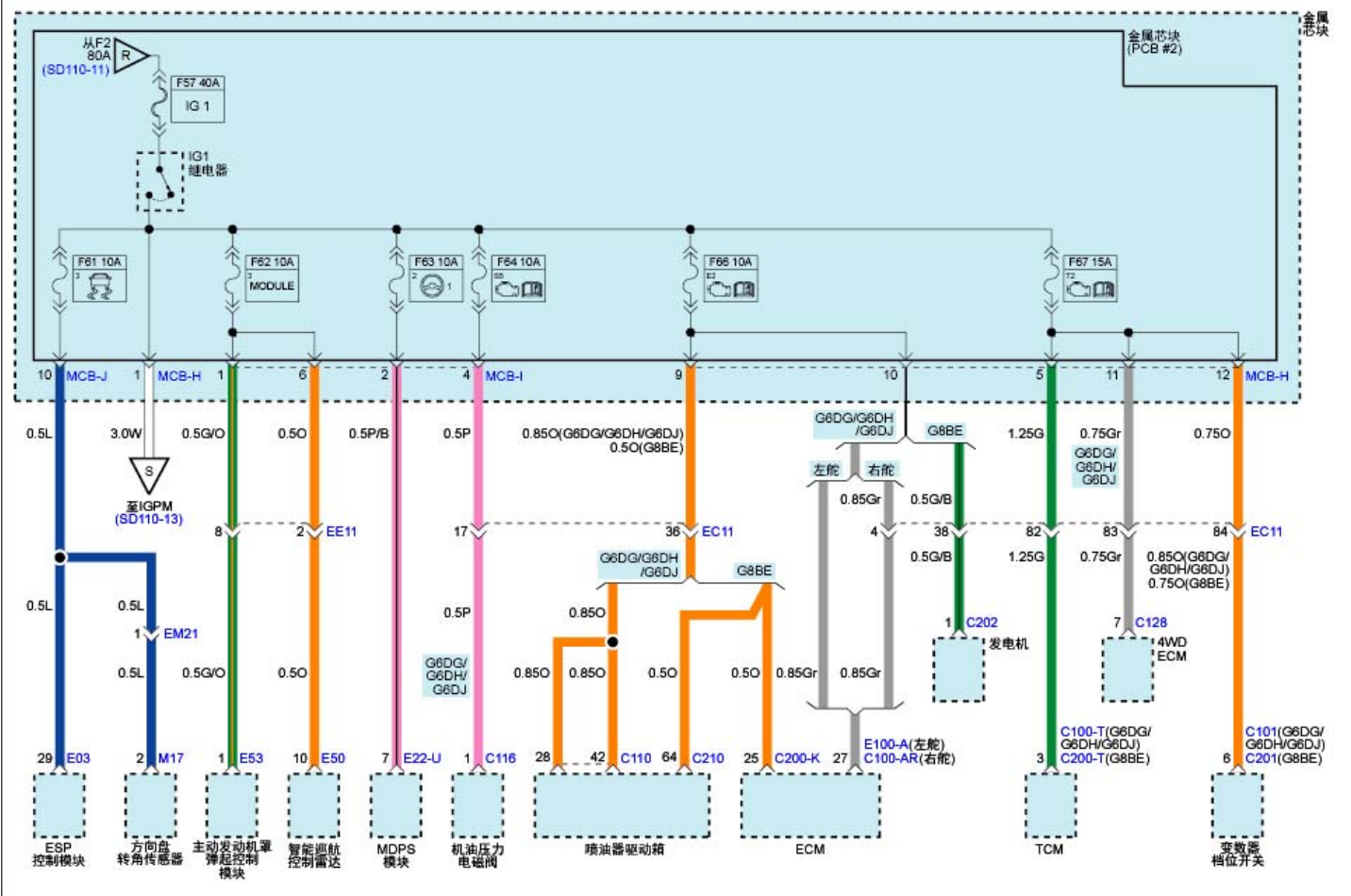
电源分布(12)
